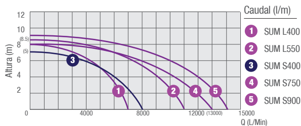
Diagrama de rendimiento (at n=2850 r.p.m.)
